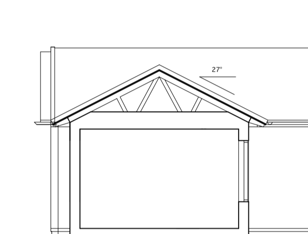
Sektion genom vinkelbyggnad
