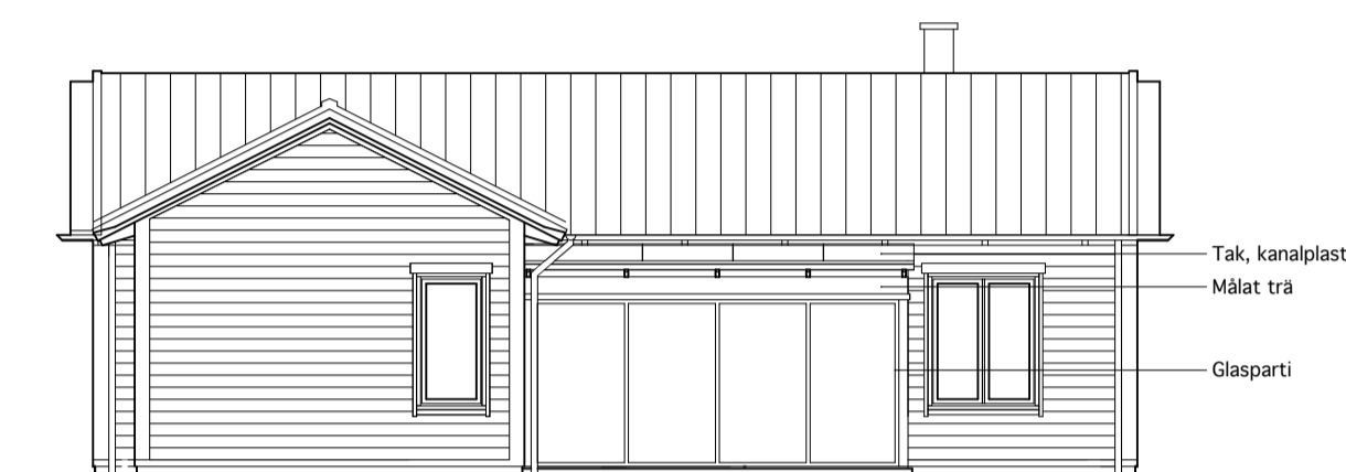
Uteplatsfasad
