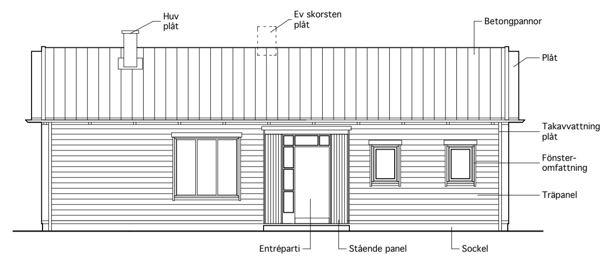
Entréfasad
