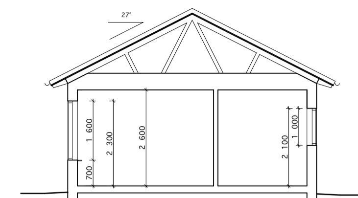
Sektion
