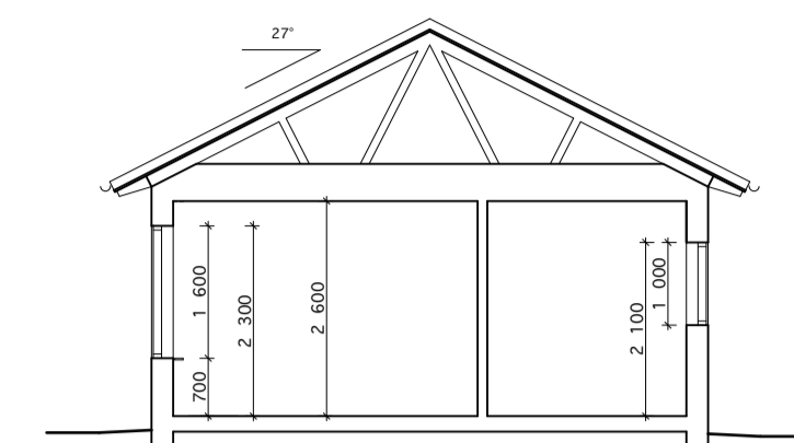
Sektion
