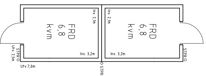
FÖRRÅD VID HUS 104, 107, 210, 213
