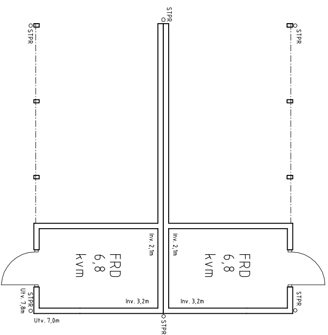
EV FRAMTIDA CARPORT VID HUS 104, 107 210, 213
